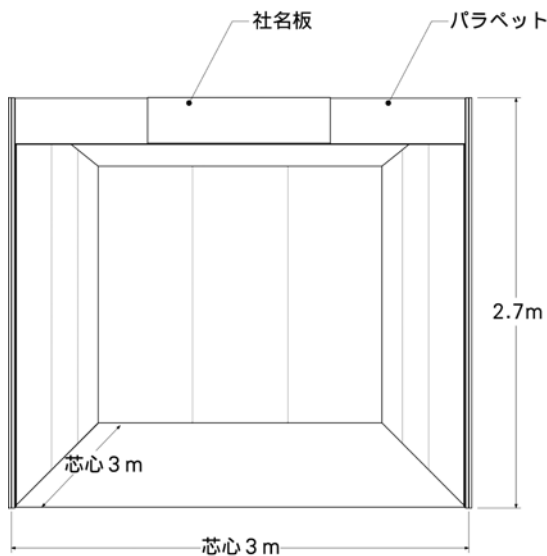
一般小間の基礎仕様 (両袖パネル+背面パネル+正面パラベット+社名板)
