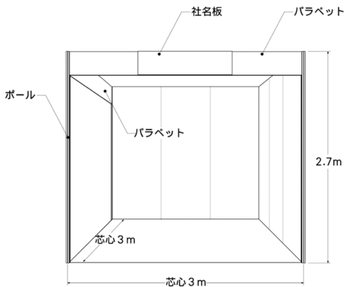
角小間の場合の一般小間 (袖パネル+背面パネル+2面パラベット+ポール+社名板)
